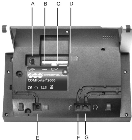
Abb. 4: Sockets
