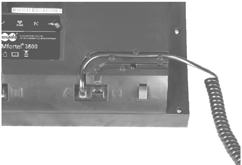
Abb. 4: Anschluss des Hörers
