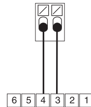
scatola di collegamento RJ-11
