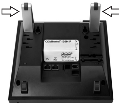
Abb. 2: Gehäusefüße
